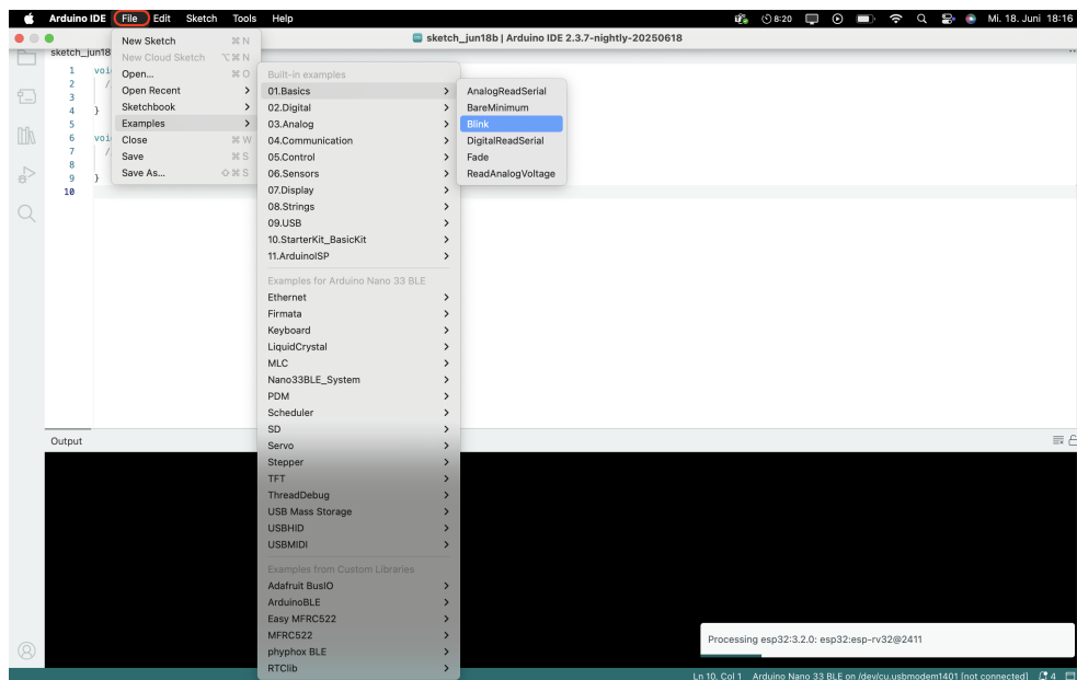
Abbildung 2.26.: Beispielprogramme öffnen
